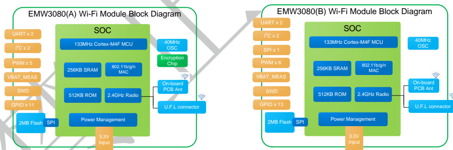
EMW3080 硬件框图模块接口
