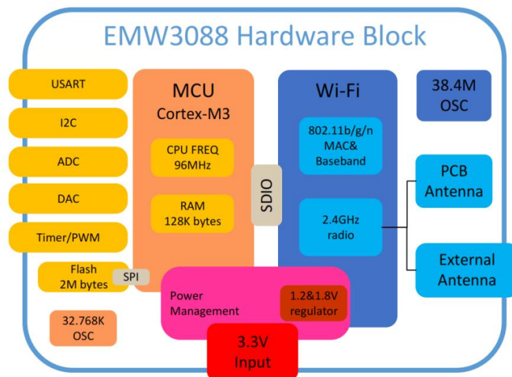
图 1 EMW3088 硬件框图模块接口
