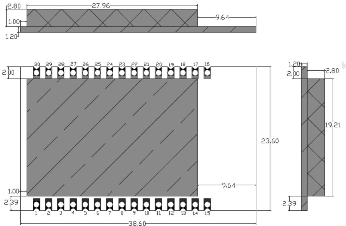
图 11 EMW3088 三视图（单位：mm）
