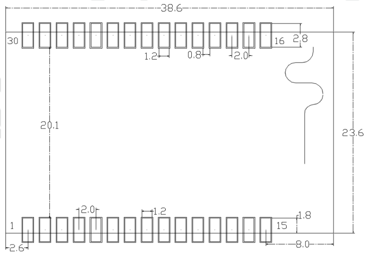
图 4 推荐邮票口封装尺寸示意图
