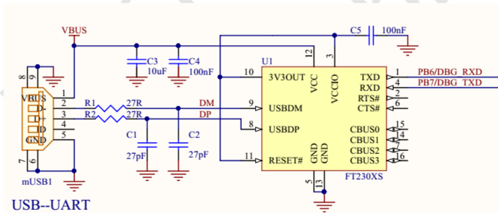
图 16 USB 转串口参考电路
