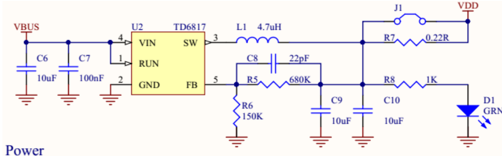
图 15 电源参考电路
