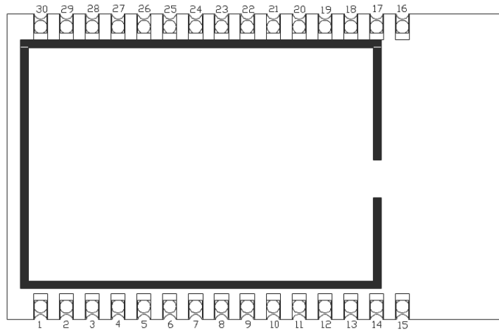
图 3 EMW3088 引脚排列示意图
