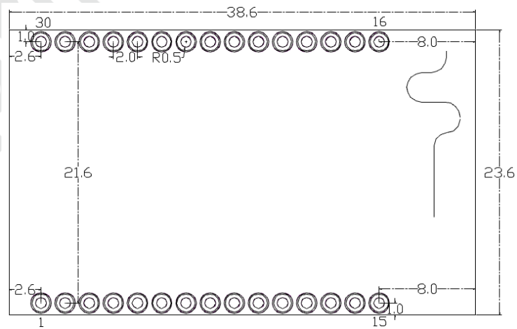
图 5 推荐 DIP 封装尺寸示意图
