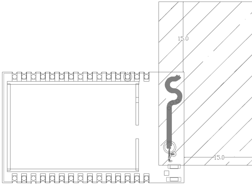
图 9 PCB 天线最小净空区 (单位: mm)
