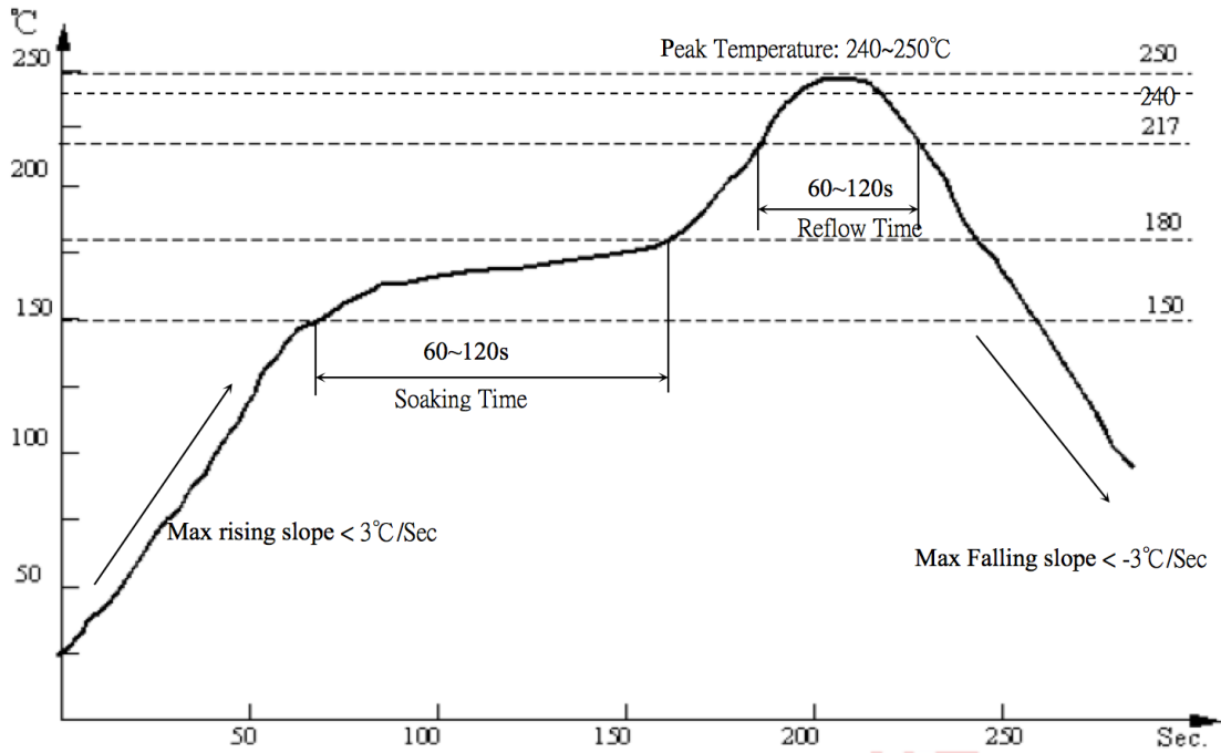
图 14 参考回流温度曲线
