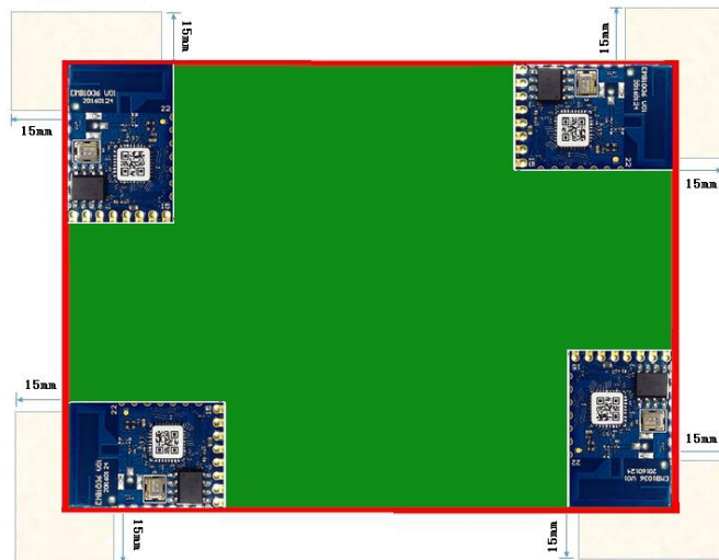
图 2.4 参考模块区域图
