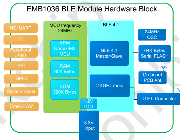
图 1.2 硬件框图
