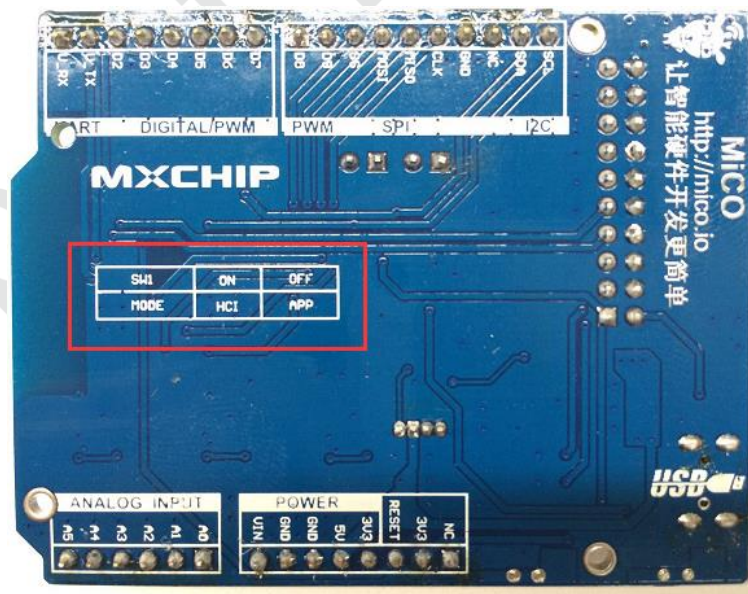
图 3.2 BLEKit-1036 背面图
