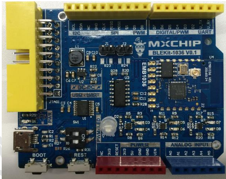
图 3.1 BLEKit-1036 正面图
